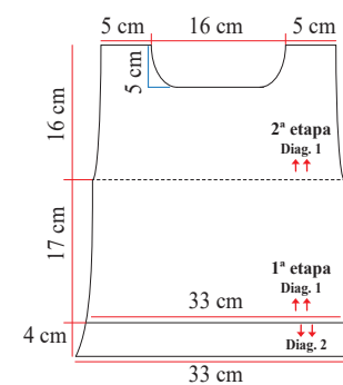
Esquema de medidas
